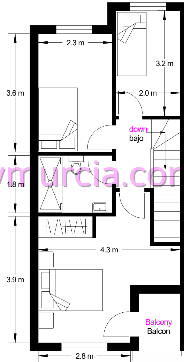
Top floor-Planta alta 47m2
